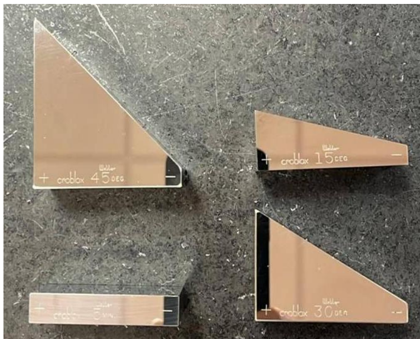
Imagen 1. Fotografía del patrón viajero: Juego de bloques patrón angulares.
